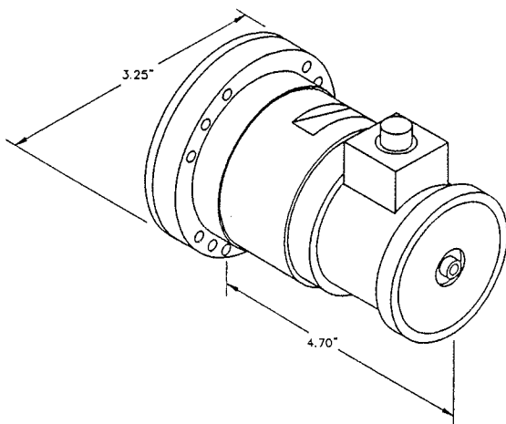
Figure 25. HBM Torsiógraph.
